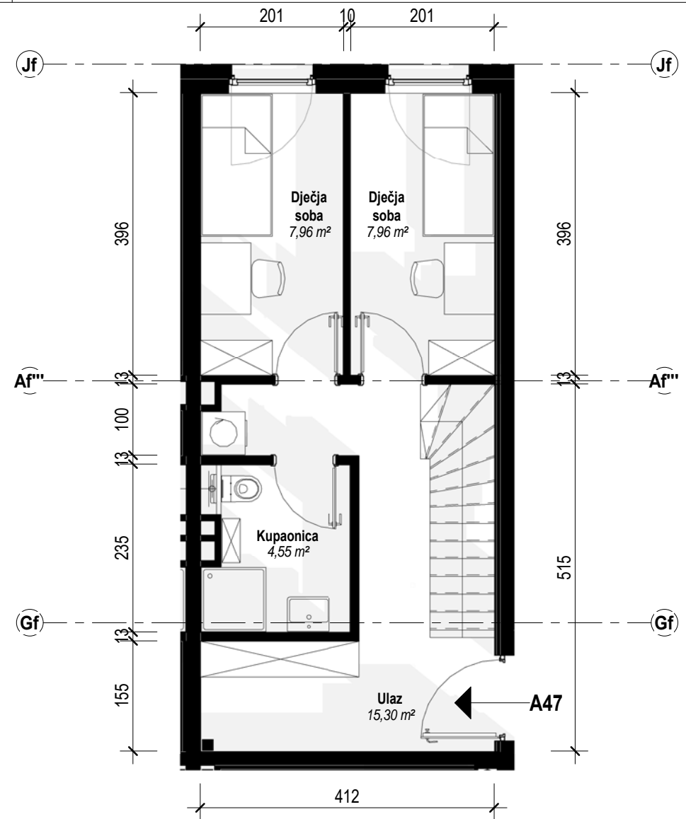
2 Level 7 (+4) - Stan A47 1 : 75
